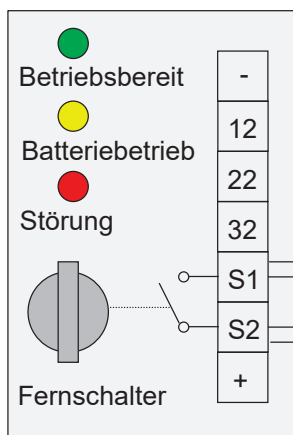
F3-Modul
