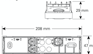
Deckeneinbau-Kit
