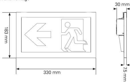
Maßangaben in mm CrystalWay 19022 CG-S
