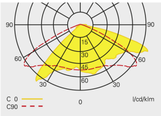
Lichtverteilungskurve Outdoor Wall II O CG-S mit symmetrischer Optik
